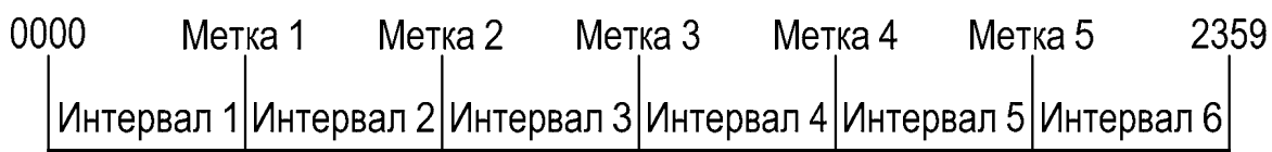
Рисунок 14 – Схема организации таймера
