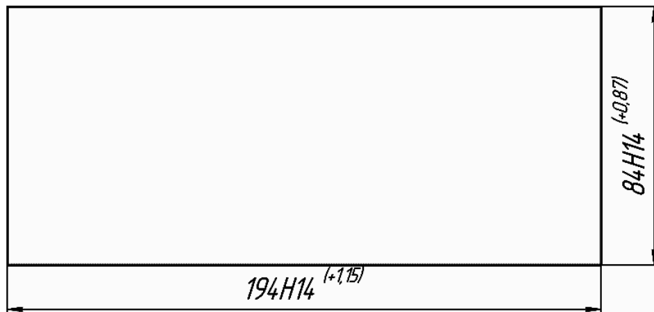
Рисунок 3 - Размеры окна в панели для крепления реле РДЦ – 06 - 2 (утопленный монтаж)
