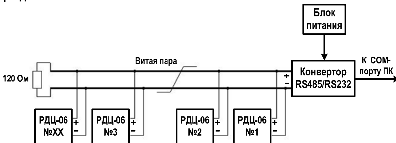
Рисунок 15 - Схема подключения реле к ПК
