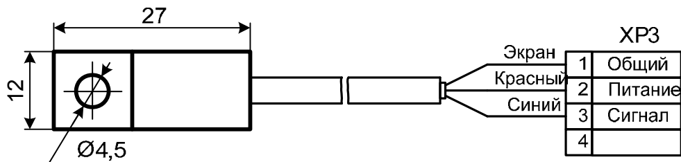
Рисунок 16 - Габаритные размеры и схема подключения датчика температуры
