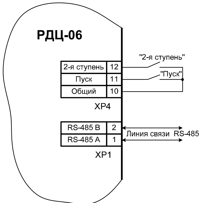
Рисунок 9 - Схема управления реле входными сигналами "Пуск" и "2-я ступень" и подключения линии связи интерфейса RS-485
