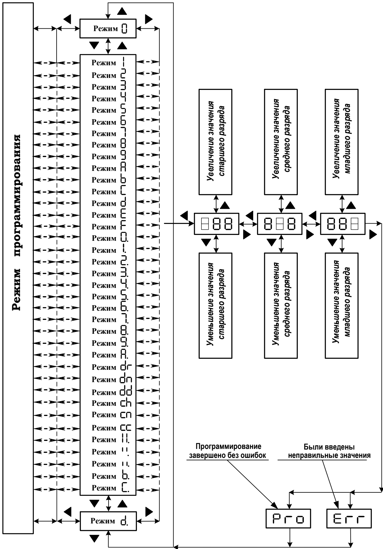
Рисунок 13 - Алгоритм работы реле в режиме программирования
