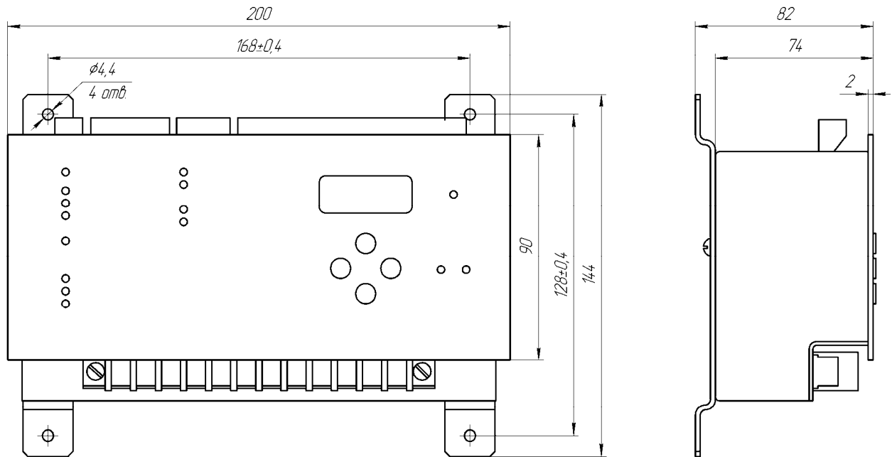
Рисунок 1 - Габаритные и установочные размеры реле РДЦ – 06 - 1 (выступающий монтаж)
