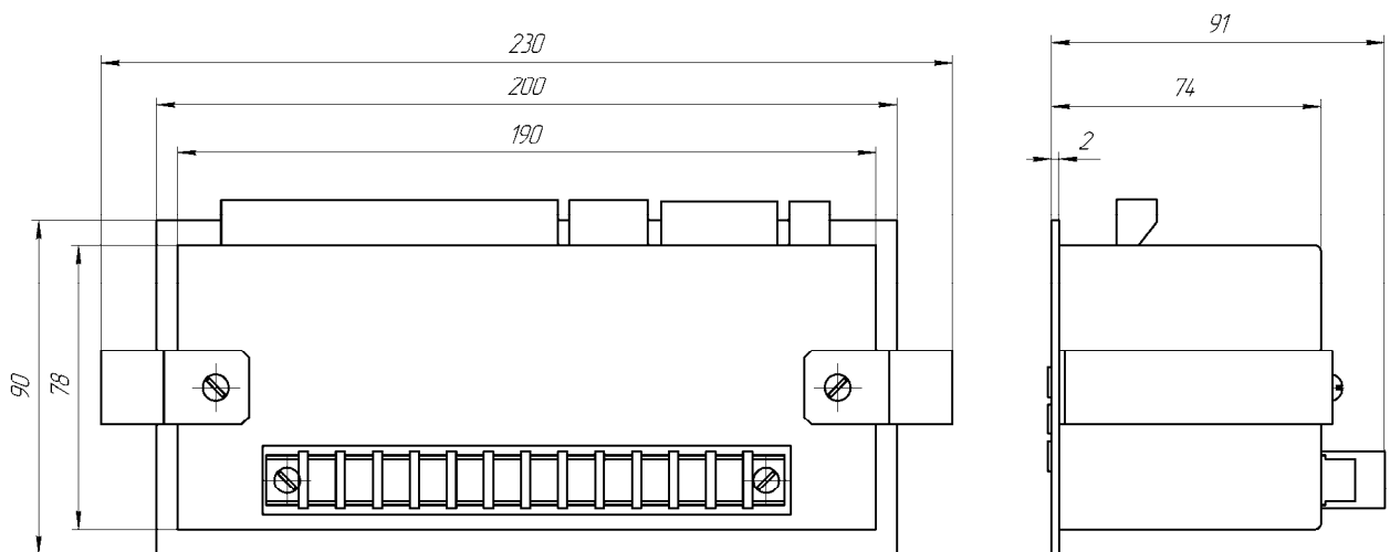
Рисунок 2 - Габаритные и установочные размеры реле РДЦ – 06 - 2 (утопленный монтаж)
