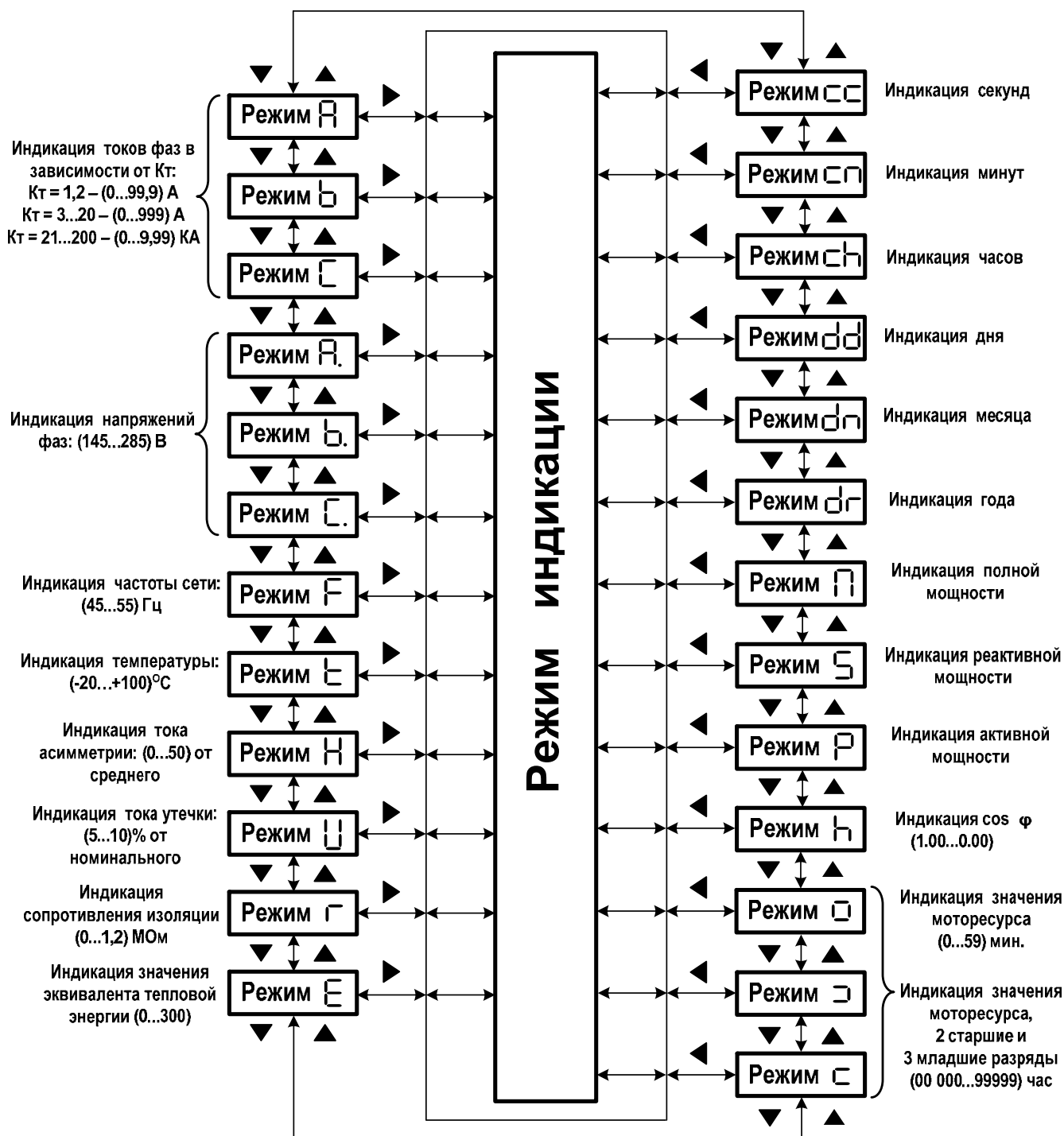
Рисунок 12 - Алгоритм работы реле в режиме индикации
