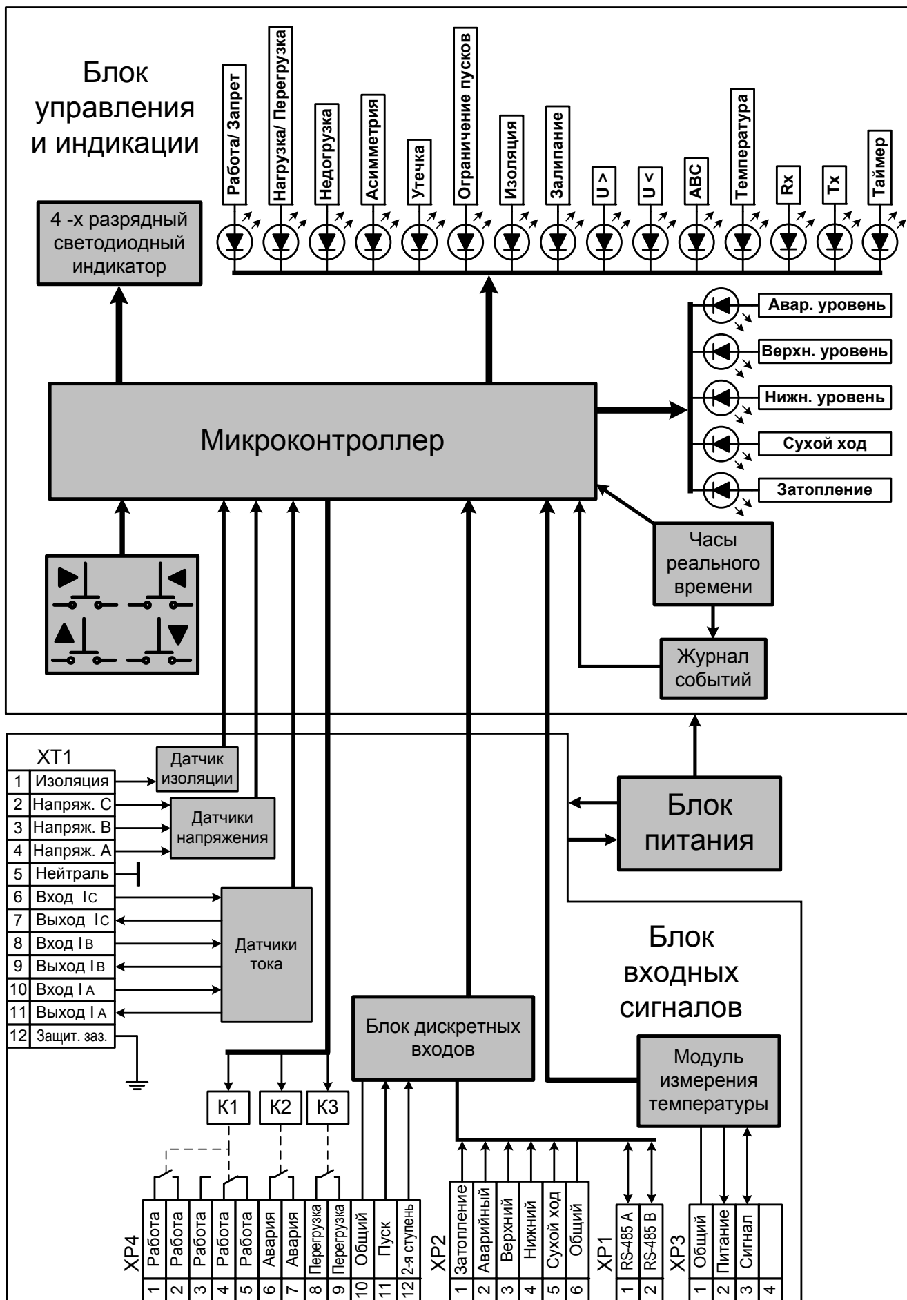
Рисунок 5 - Структурная схема реле
