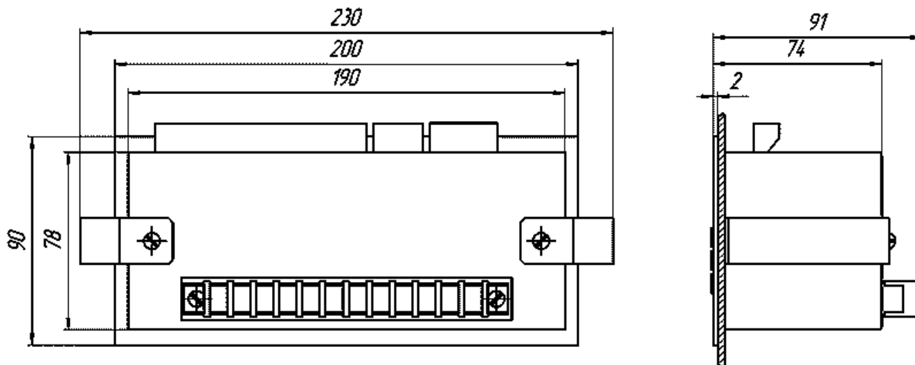
Рисунок 2 - Габаритные и установочные размеры реле РДЦ – 05 - 2 (утопленный монтаж).
