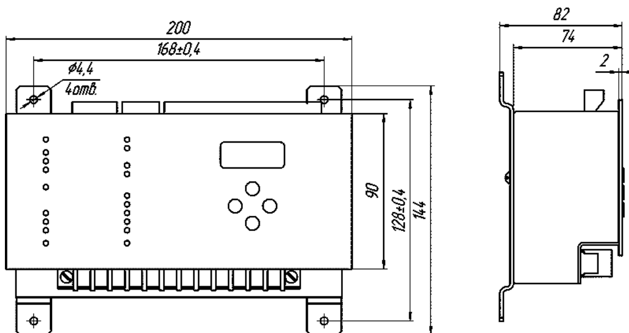
Рисунок 1 - Габаритные и установочные размеры реле РДЦ – 05 -1 (выступающий монтаж).
