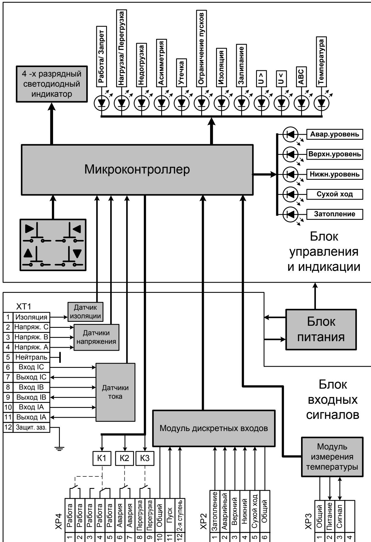
Рисунок 5 - Структурная схема реле защиты электродвигателя РДЦ-05.
