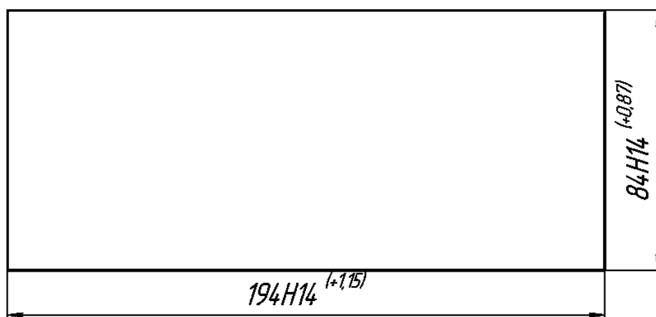
Рисунок 3 - Размеры выреза в панели для крепления реле РДЦ – 05 - 2 под утопленный монтаж
