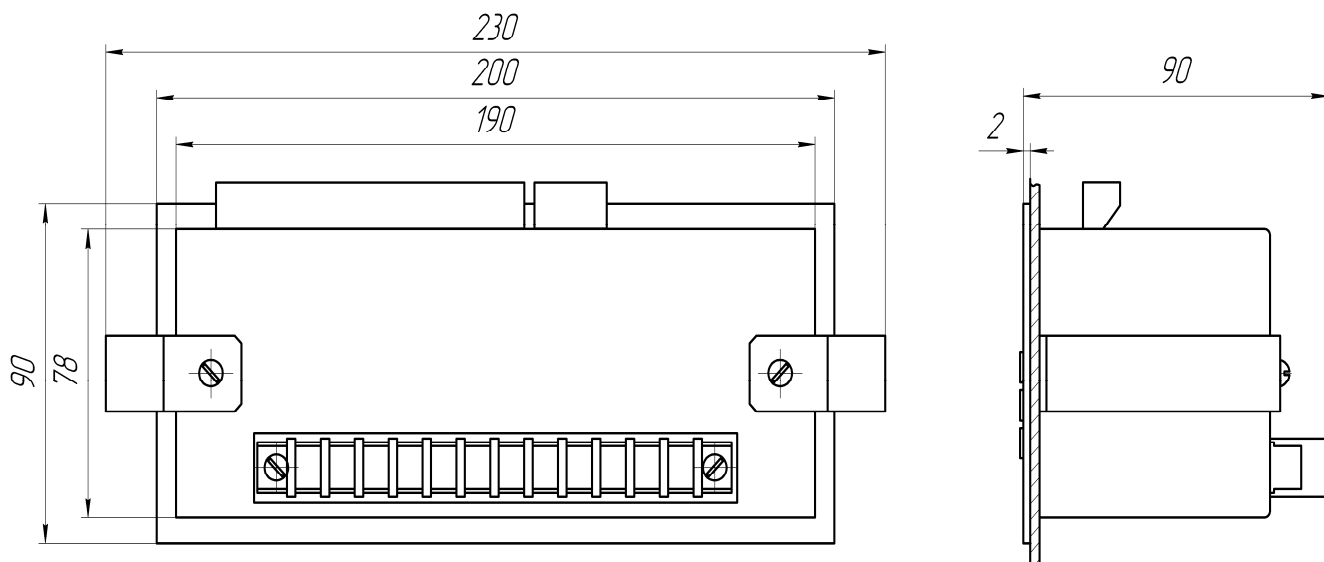
Рисунок 2 - Габаритные и установочные размеры реле РДЦ – 03 -2 (утопленный монтаж).
