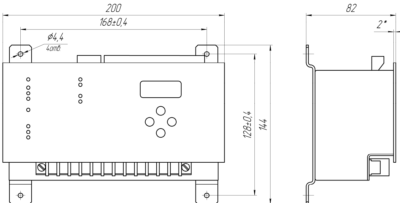
Рисунок 1 - Габаритные и установочные размеры реле РДЦ – 03 -1 (выступающий монтаж).
