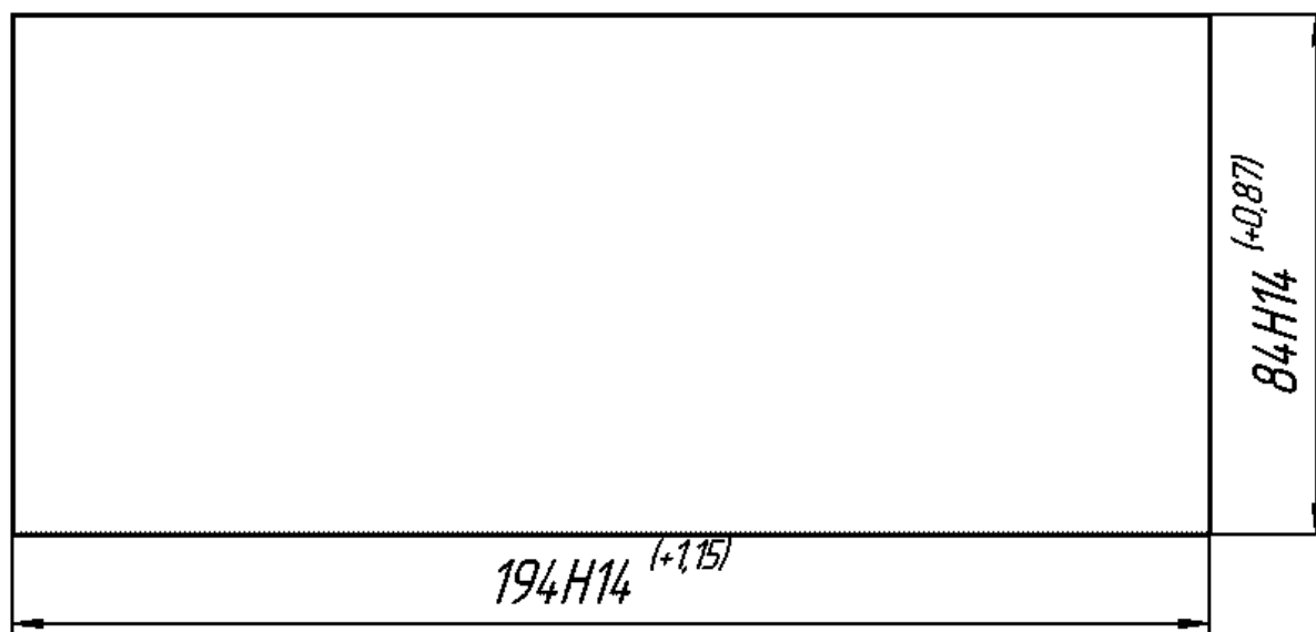
Рисунок 3 - Размеры выреза в панели для крепления реле РДЦ – 03 -2 под утопленный монтаж
