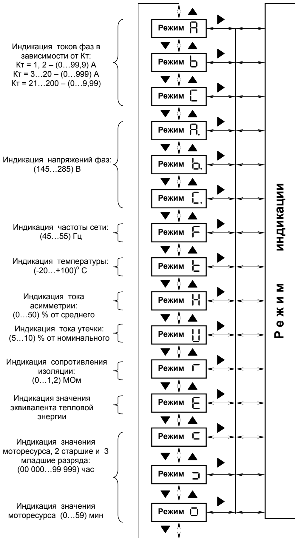
Рисунок 10 - Алгоритм работы реле РДЦ-03 в режиме индикации
