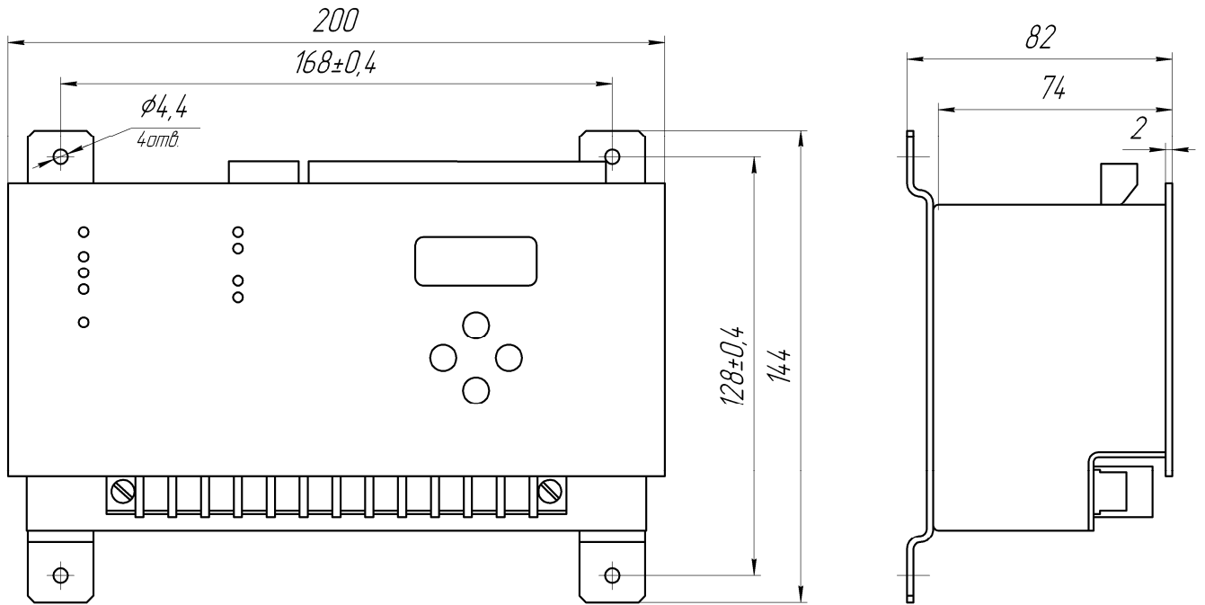
Рисунок 1 - Габаритные и установочные размеры реле РДЦ – 02 - 1 (выступающий монтаж)
