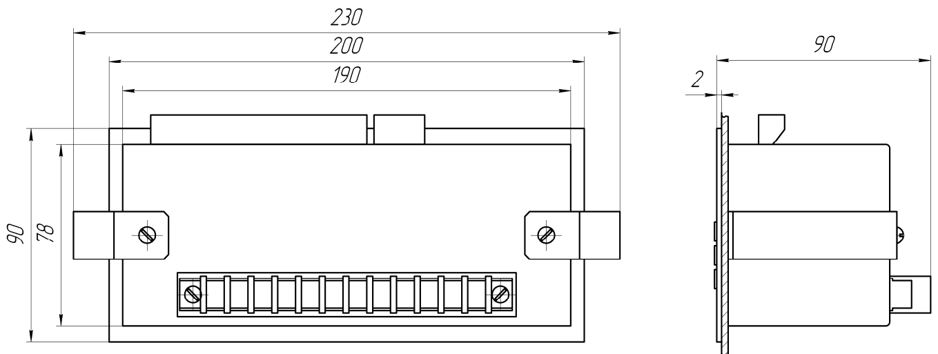
Рисунок 2 - Габаритные и установочные размеры реле РДЦ – 02 - 2 (утопленный монтаж)
