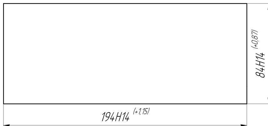
Рисунок 3 - Размеры окна в панели для крепления реле РДЦ – 02 - 2 (утопленный монтаж)
